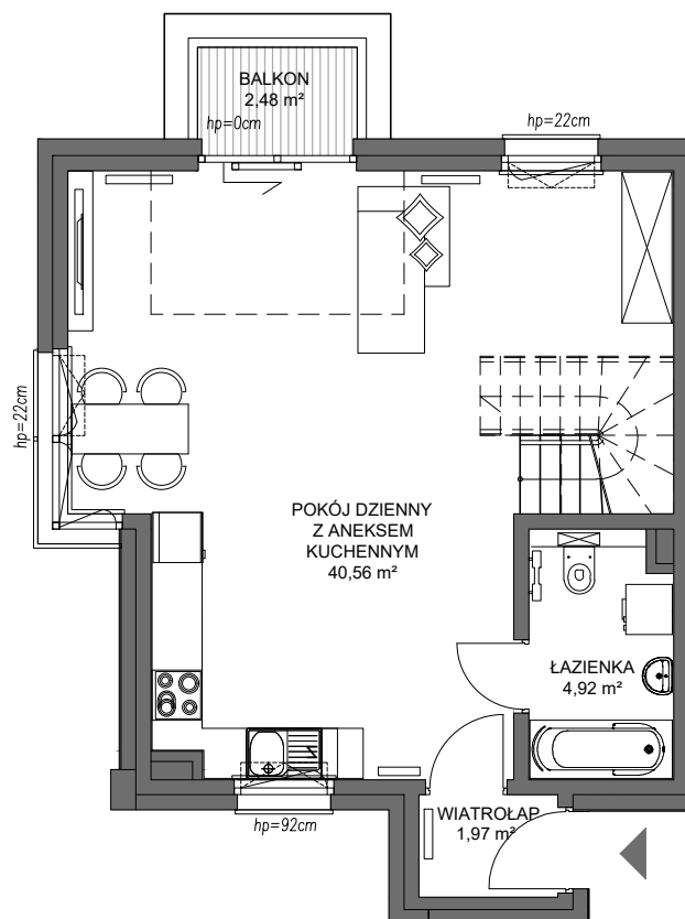
POZIOM 1
