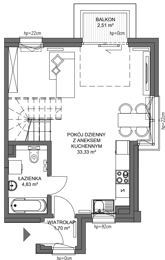
POZIOM 1
